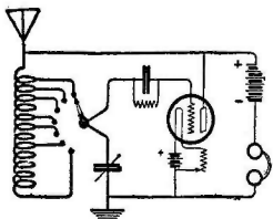
Figura N° 1.—El Regenerativo Automático con puntos. La bobina tiene 60 vueltas con un "tap" o deriva cada 10 vueltas.
