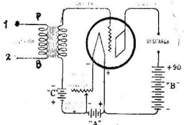
Figura N° 6.—Para obtener una reproducción natural úsese una Batería "C" como se muestra arriba, especialmente cuando se trata de ondas fuertes y de altos voltajes en la placa.
