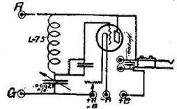
Figura N° 2.—El Regenerativo Automático sin puntos.
