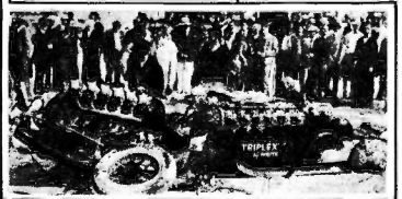
Estado en que quedó el "Triplex" después del accidente sufrido a una velocidad de 202 millas por hora. (Fotos Underwood & Underwood).
