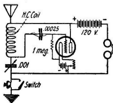
Figura N° 3.—El Regenerativo Automático, convertido en transmisor, un micrófono, en tierra, y 120 volts en la placa. Las alteraciones en el resto del circuito son bien leves. Compare los circuitos.
